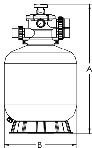
RO-400N-VT/ 525 / 625
