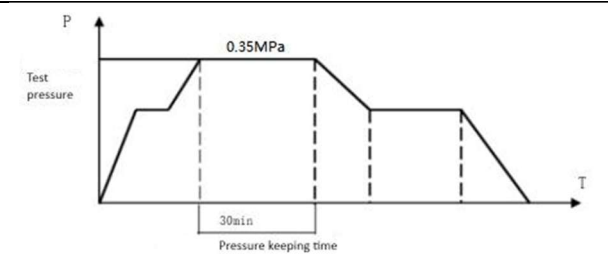
Actual pressure test curve
