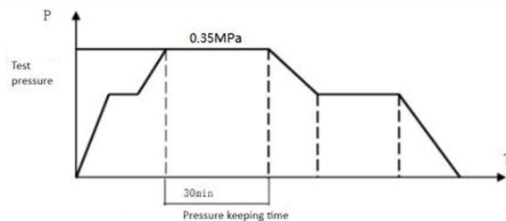
Actual pressure test curve
