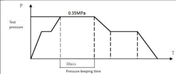
Actual pressure test curve
