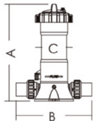
CL-300F, CL-400F
