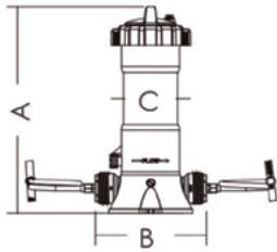
CL-320F, CL-420F
