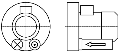
Fig. 1: Turbinas de canal lateral de simple etapa (1 rodete) Single stage side channel blower (1 impeller) Soufflante mono-étagée à canal latéral (1 roue à aubes) Series: ASC/ARBxxx-1M...
